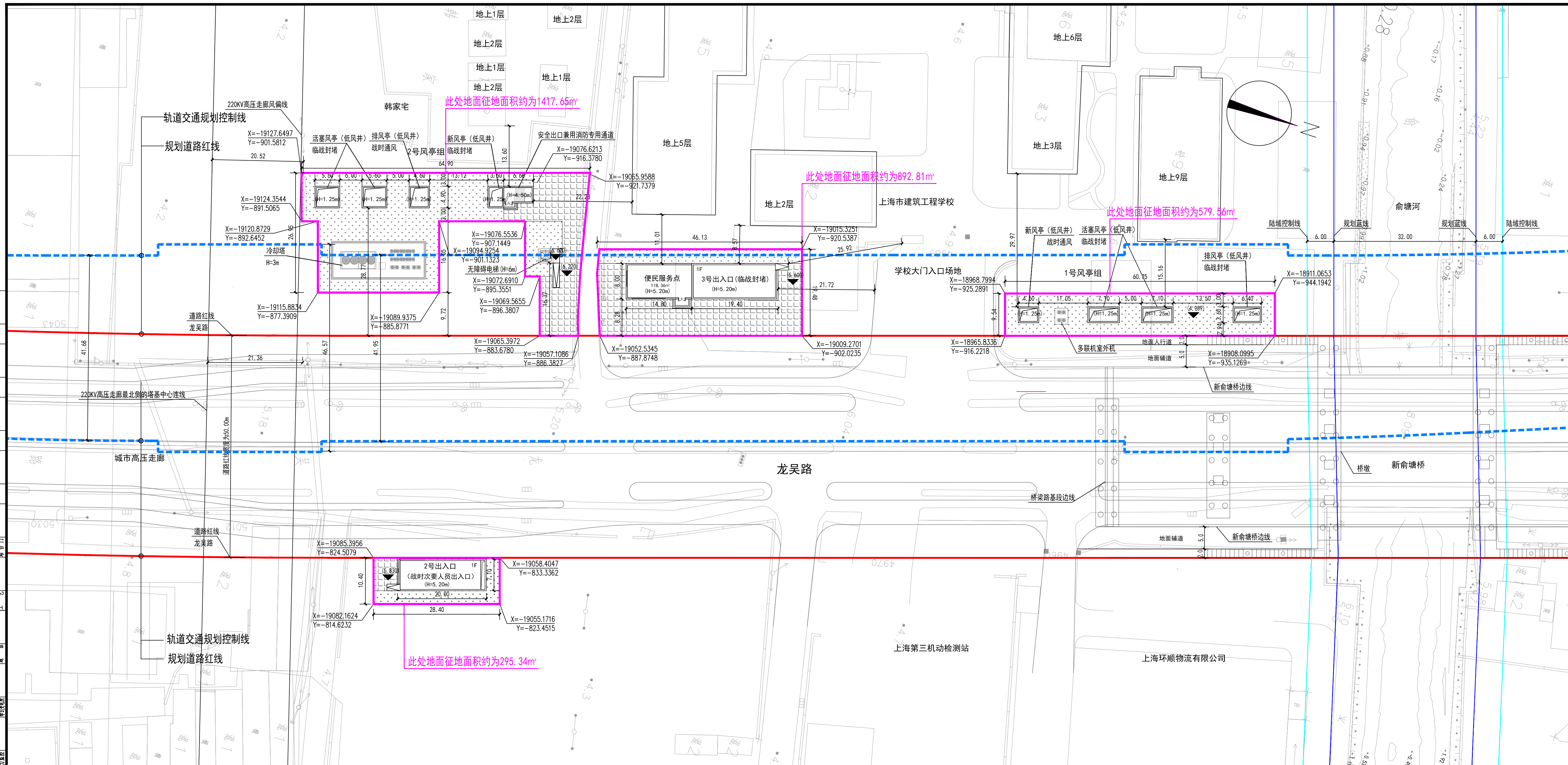
总平面图 1:500
